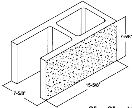
8" x 8" x 16" ** S1S OE1E
