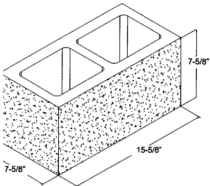
8" x 8" x 16" S1S1E
