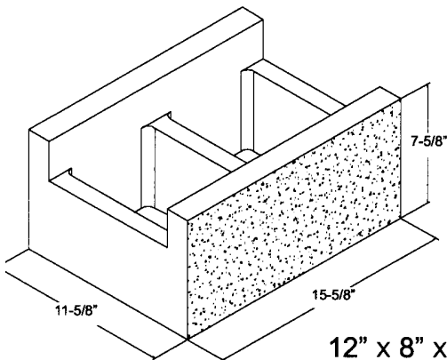
12" x 8" x 16" ** S1S1E
