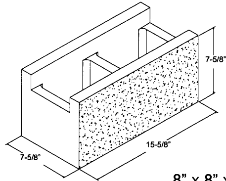
8" x 8" x 16" ** S1S DCBB
