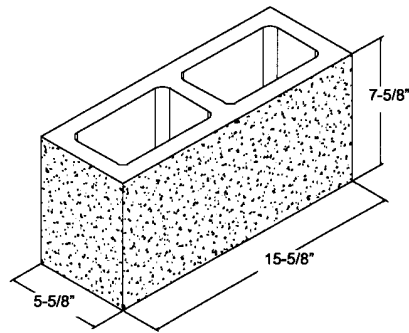
6" x 8" x 16" ** S1S1E
