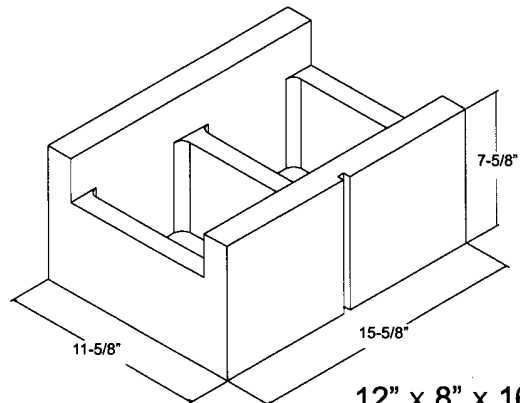
12" x 8" x 16" ** DCBB
