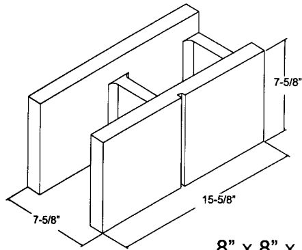
8" x 8" x 16" ** DCBB OE1E
