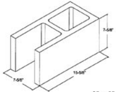
8" x 8" x 16" OE1E
