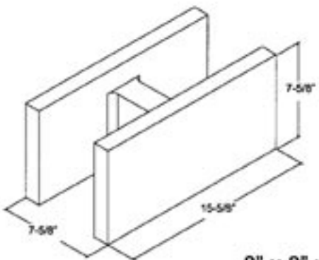
8" x 8" x 16" ** CBB OE2E
