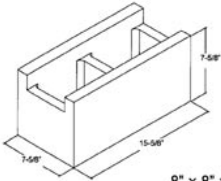
8" x 8" x 16" DCBB
