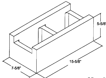
8" x 6" x 16" CBB
