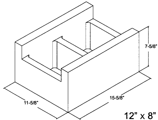
12" x 8" x 16" ** OE1E
