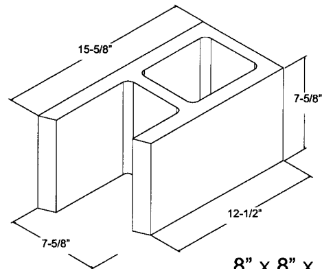
8" x 8" x 16" 45° ANGLE
