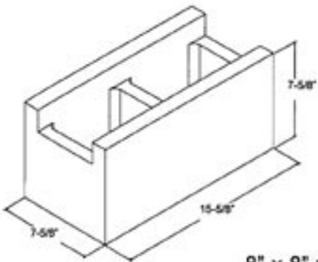
8" x 8" x 16" SBBB
