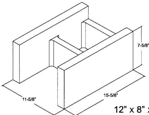
12" x 8" x 16" DCBB
