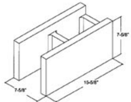
8" x 8" x 16" DCBB OE1E
