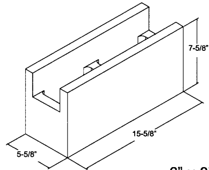
6" x 8" x 16" DCBB
